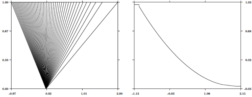
FIGURA 6.7. Ejemplo 6.11 (ecuaciones shallow water , continuación: problema dam break (rotura de la presa)): la solución del problema en el espacio (x, t) (izquierda) y la componente h (derecha).
