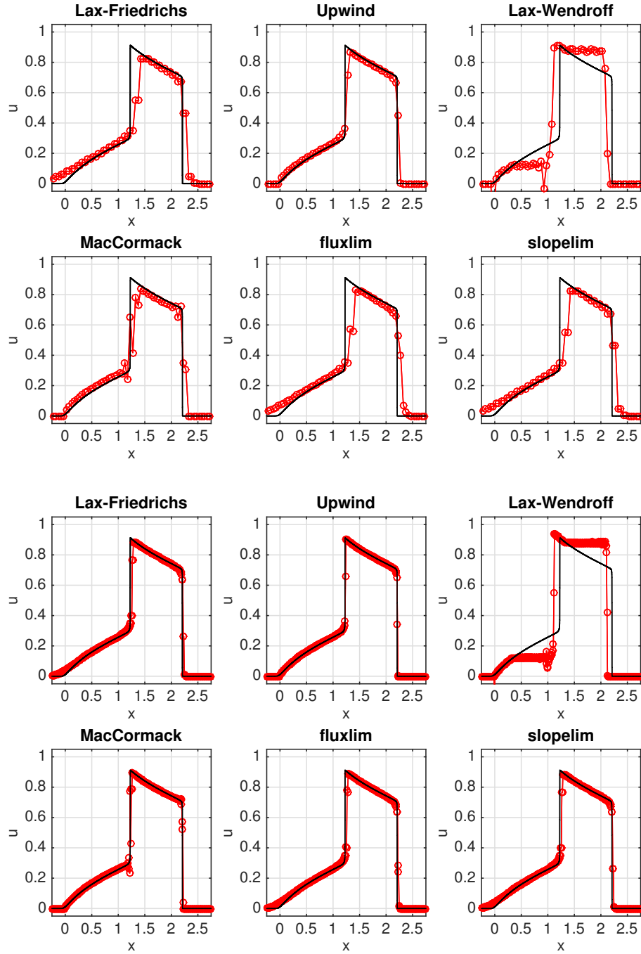
FIGURA 4.6. Ejemplo 4.3: solución numérica de la ecuación de Buckley-Leverett con u_0 dada por (4.17). Arriba: \Delta x = 1/20 ; abajo: \Delta x = 1/100 . La línea sólida es la solución de referencia.
