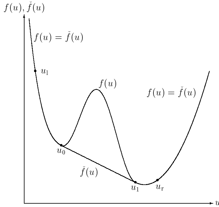
FIGURA 3.2. La función f(u) y su envoltura convexa inferior \check{f}(u) para los valores de u_1 y u_r . Las funciones f(u) y \check{f}(u) coinciden para u_1 \leq u \leq u_0 y u_1 \leq u \leq u_r .
