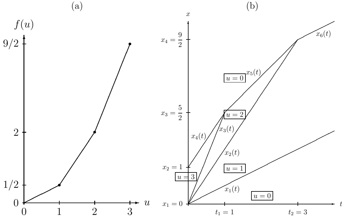
FIGURA 3.5. Ejemplo 3.2: (a) grafo de f , (b) solución global del problema.
