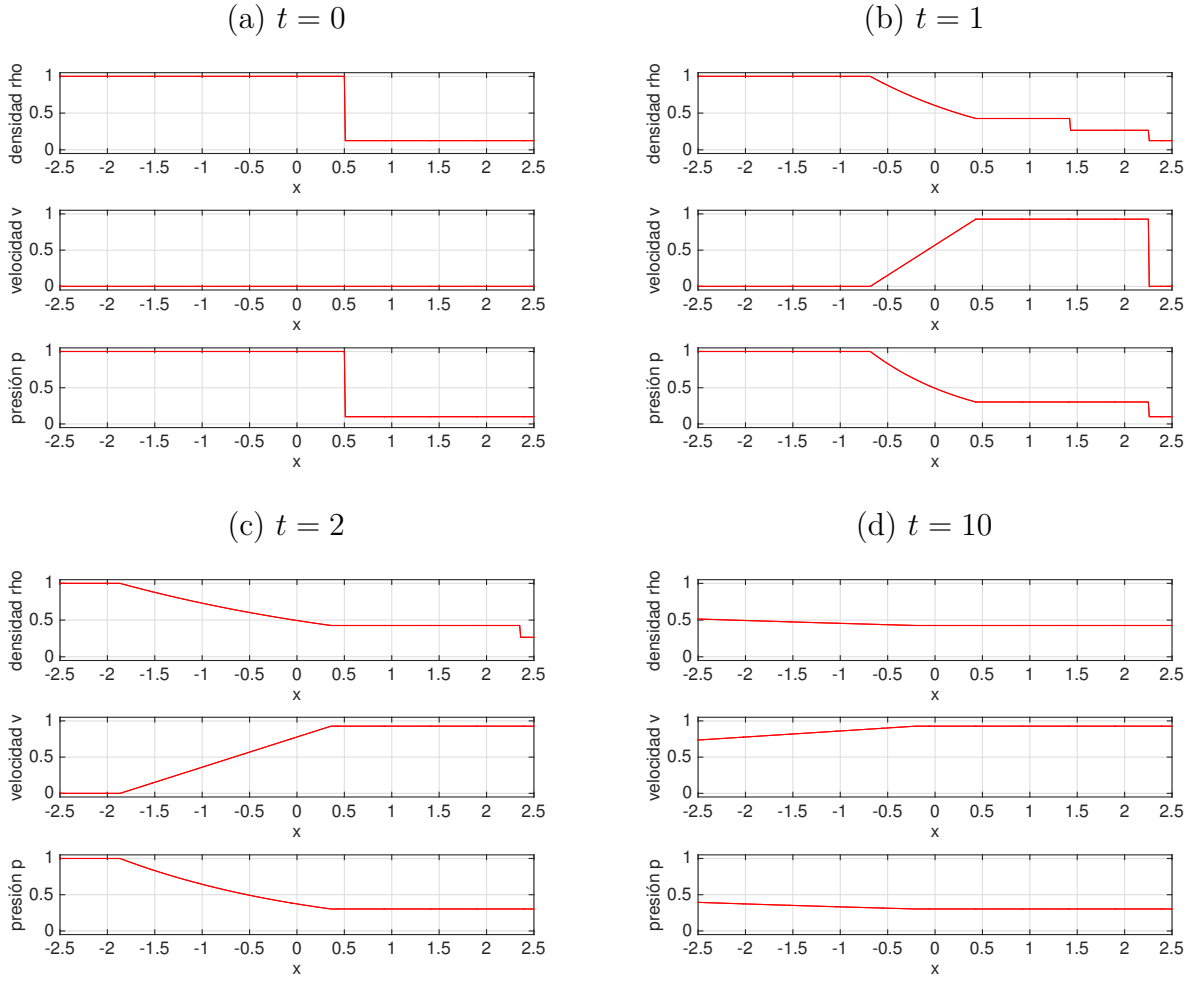
FIGURA 6.9. Ejemplo 6.12 (ecuaciones de Euler, problema de Sod): (a) dato inicial (6.101) , (b–c) solución (6.106) para \rho , v , y p en los tiempos indicados.
