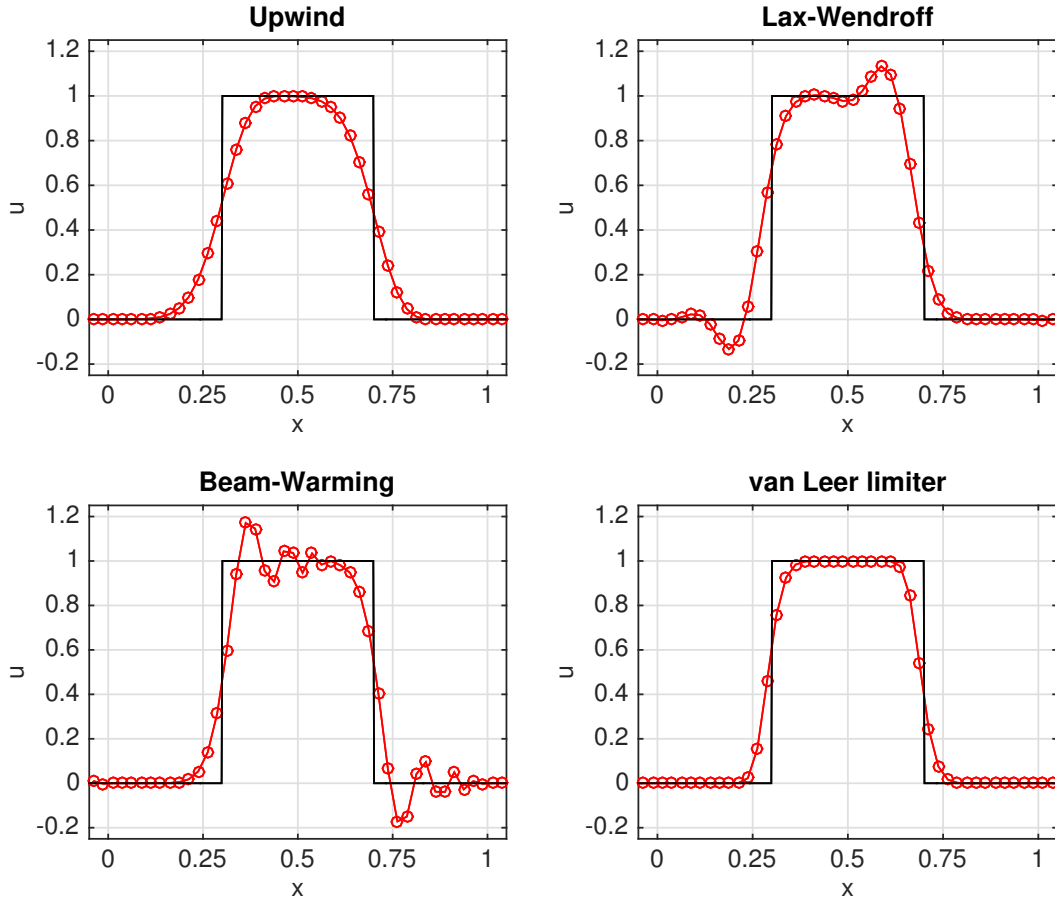
FIGURA 4.9. Ejemplo 4.7: solución numérica de la ecuación de transporte por los métodos upwind , de Lax-Wendroff, de Beam-Warming, y el método (4.31) basado en el limiter de van Leer (4.35).
