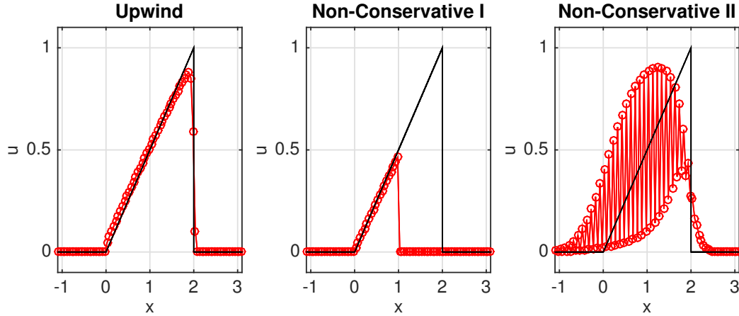
FIGURA 4.1. Ejemplo 4.1: (izquierda) Solución de entropía de la ecuación de Burgers (línea sólida, trazada en los tres plots) con aproximación por un método conservativo (método upwind ), (centro) aproximación por el método no conservativo (4.7), (derecha) aproximación por el método no conservativo (4.9). En cada caso, \Delta x = 1/20 , \lambda = 1/2 .
