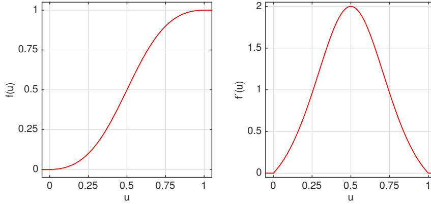
FIGURA 4.4. Ejemplo 4.3: (izquierda) la función f(u) definida por (4.13), (derecha) su derivada f'(u) (4.14).
