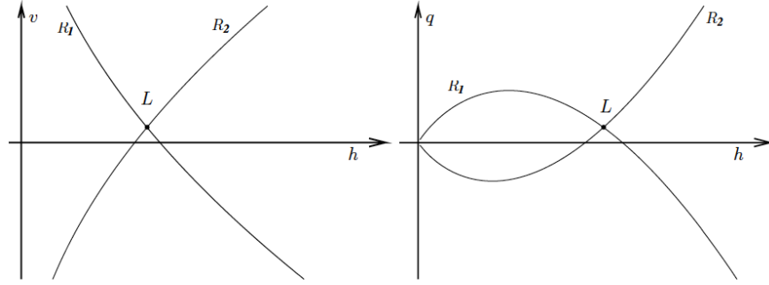
FIGURA 6.2. Ejemplo 6.6 (ecuaciones shallow water : ondas de rarefacción): curvas de rarefacción en los planos (h, v) (izquierda) y (h, q) (derecha). Se ilustra la solución completa (6.18) para las ecuaciones shallow water . Solamente las partes dadas por (6.26) y (6.27) efectivamente serán curvas de rarefacción.
