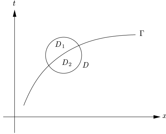
FIGURA 2.3. La derivación de la condición de Rankine-Hugoniot.
