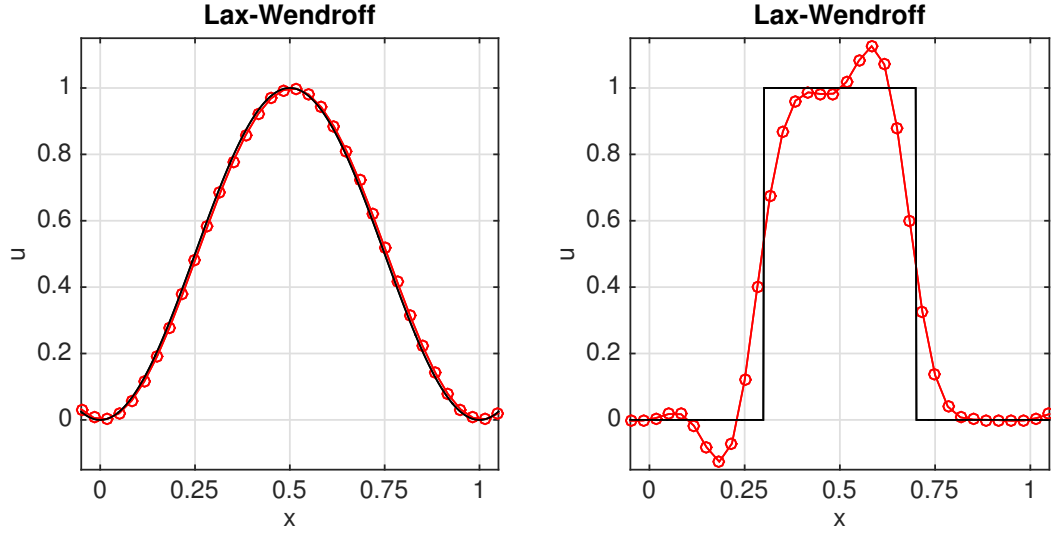
FIGURA 4.7. Ejemplo 4.6: solución de la ecuación de transporte u_t + u_x = 0 con el método de Lax-Wendroff con dato inicial (izquierda) suave, (derecha) discontinuo constante a trozos.
