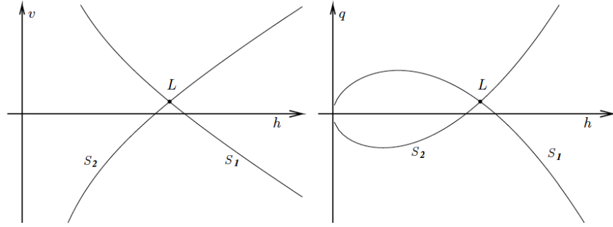
FIGURA 6.3. Ejemplo 6.7 (ecuaciones shallow water : curvas de choque): curvas de choque en los planos (h, v) (izquierda) y (h, q) (derecha). Se indican los choques lentos ( S_1 ) y rápidos ( S_2 ) (ver (6.60) y (6.61), respectivamente).
