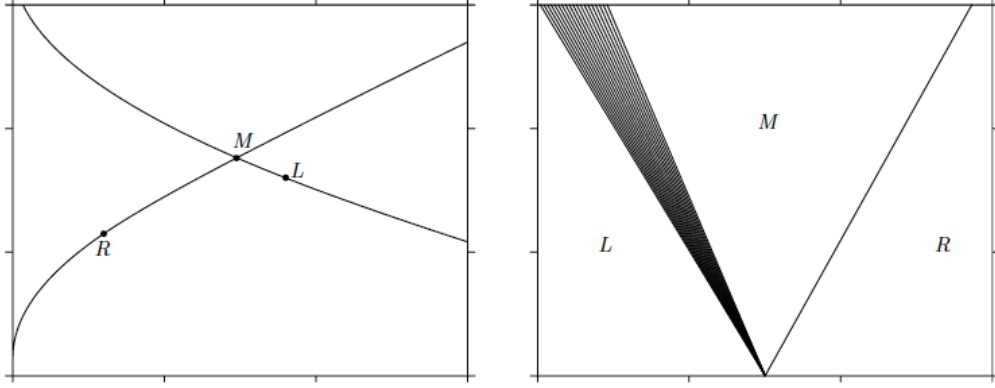
FIGURA 6.6. Ejemplo 6.9 (ecuaciones shallow water , continuación: solución del Problema de Riemann): la solución del problema de Riemann en el espacio de fase (izquierda) y en el espacio (x, t) (derecha).
