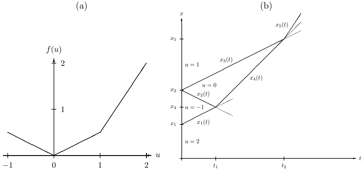
FIGURA 3.3. Ejemplo 3.1: (a) la función de flujo f(u) continua y lineal por trozos, (b) la solución constante por trozos.
