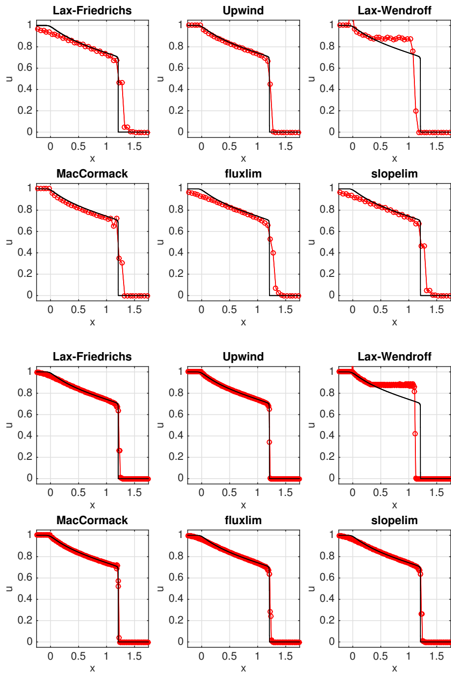
FIGURA 4.5. Ejemplo 4.3: solución numérica de la ecuación de Buckley-Leverett con u_0 dada por (4.15). Arriba: \Delta x = 1/20 ; abajo: \Delta x = 1/100 . La línea sólida es la solución de referencia.
