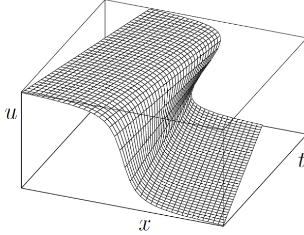
FIGURA 2.1. Ejemplo 2.5 (Ecuación de Burgers): superficie en el espacio (t, x, u) parametrizada por (2.12), u_0(x) = -\arctan x [26].
