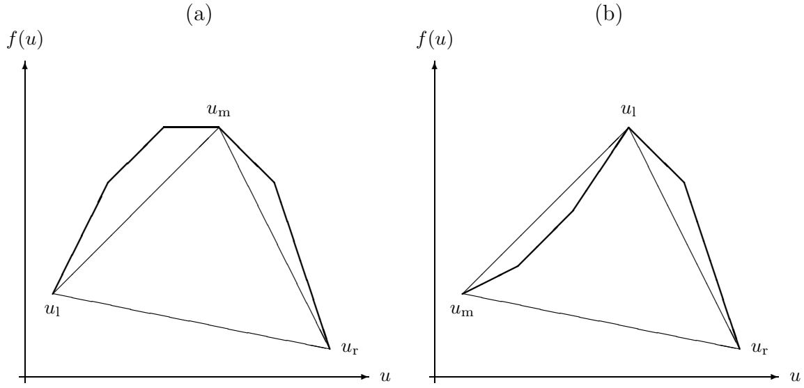
FIGURA 3.4. Demostración del Lema 3.4: (a) el caso u_l < u_l < u_r , (b) el caso u_m < u_m < u_r .
