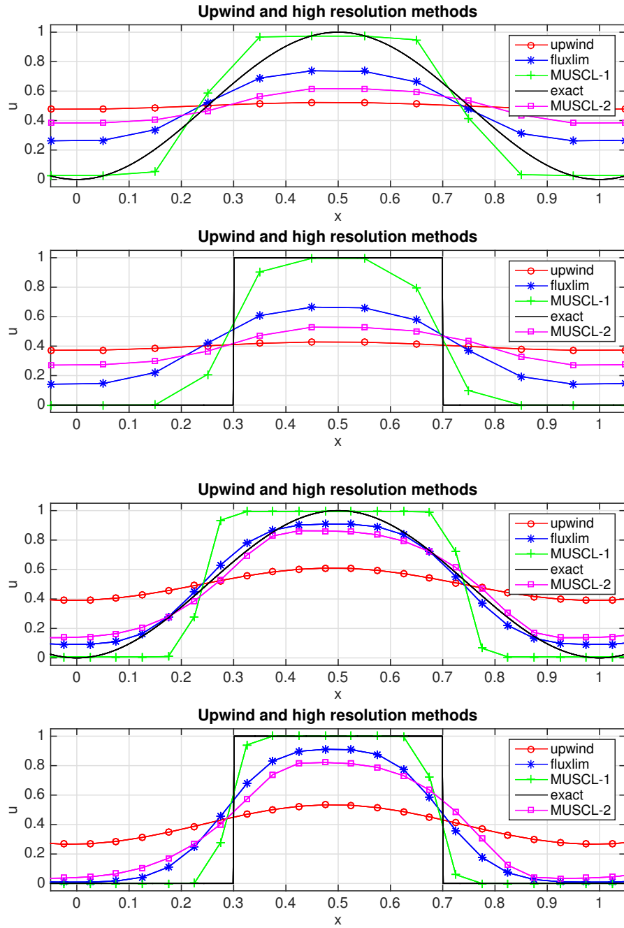
FIGURA 4.11. Ejemplo 4.9: soluciones numéricas para \Delta x = 1/10 (arriba) y \Delta x = 1/20 (abajo).
