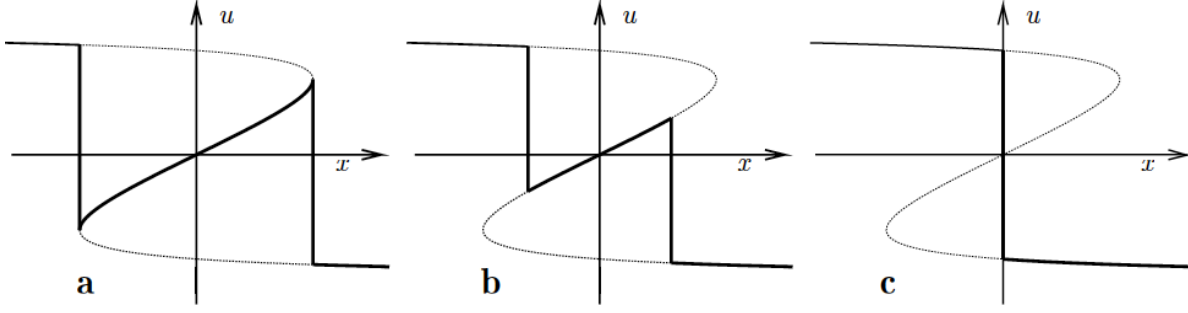
FIGURA 2.2. Ejemplo 2.6 (Ecuación de Burgers): varias soluciones u(\cdot, 3) para u_0(x) = -\arctan x con conservación de u [26].
