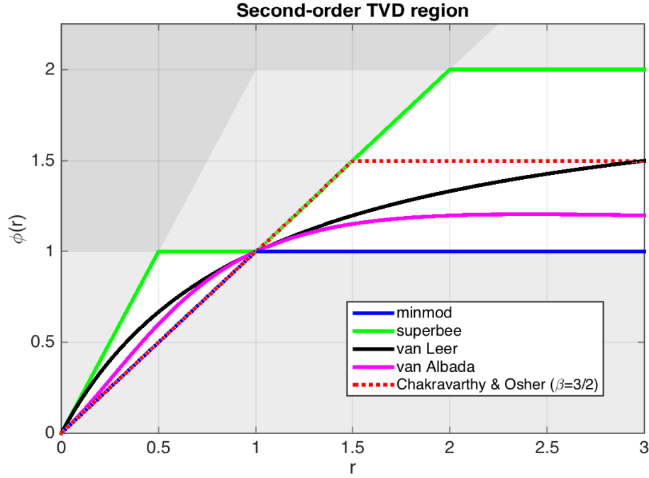
FIGURA 4.8. Grafos de funciones limiter \phi = \phi(r) . El grafo debe pertenecer a la región blanca, en la cual ambas condiciones, tanto (4.30) como (4.32), están satisfechas. En la región gris claro solamente una de las condiciones está satisfecha; en la zona gris oscuro ninguna.
