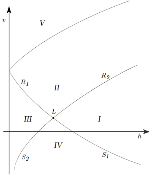
FIGURA 6.5. Ejemplo 6.9 (ecuaciones shallow water , continuación: solución del Problema de Riemann): partición del plano (h, v) , ver (6.64) y (6.71).
