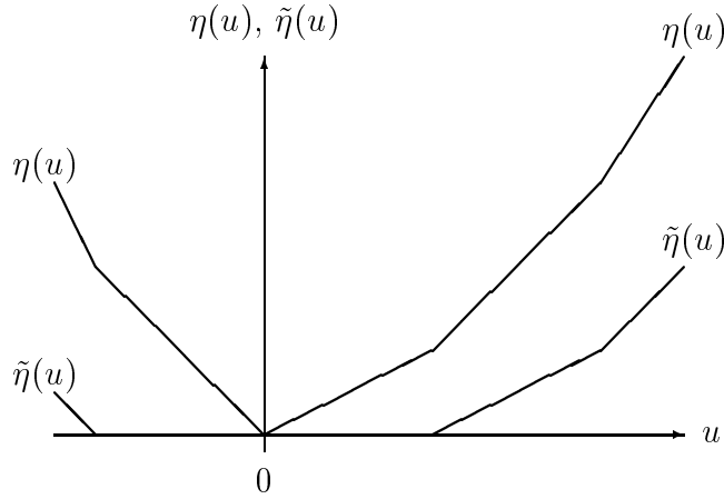
FIGURA 3.1. Demostración del Lema 3.2: las funciones \eta(u) y \tilde{\eta}(u) (ecuación (3.17)).
