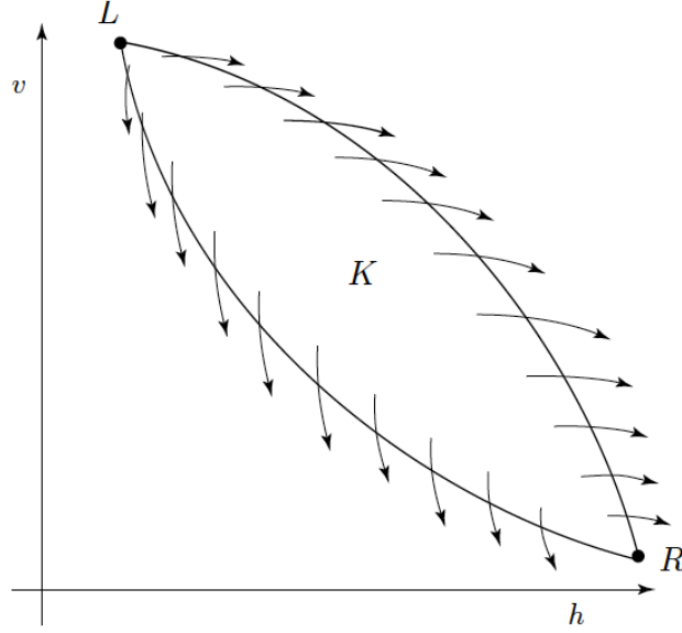
FIGURA 6.4. Ejemplo 6.8 (ecuaciones shallow water , continuación: admisibilidad de choques): el campo vectorial \mathbf{b} .
