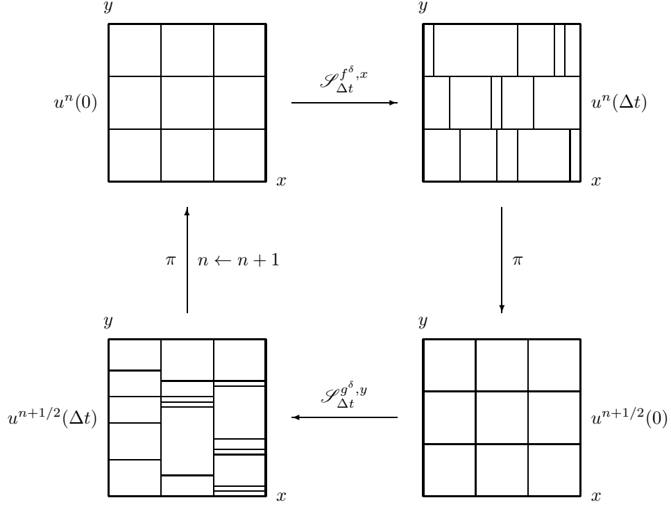
FIGURA 5.1. Splitting por dimensiones y Front Tracking para una malla 3 \times 3 .
