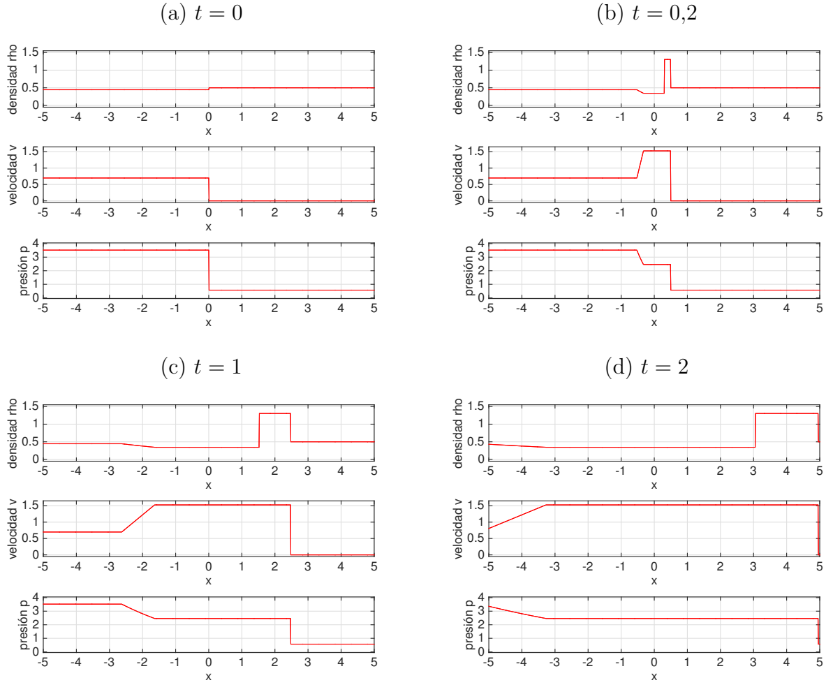
FIGURA 6.10. Ejemplo 6.13 (ecuaciones de Euler, problema de Lax): (a) dato inicial (6.107) , (b–c) solución (6.106) para \varrho , v , y p en los tiempos indicados.
