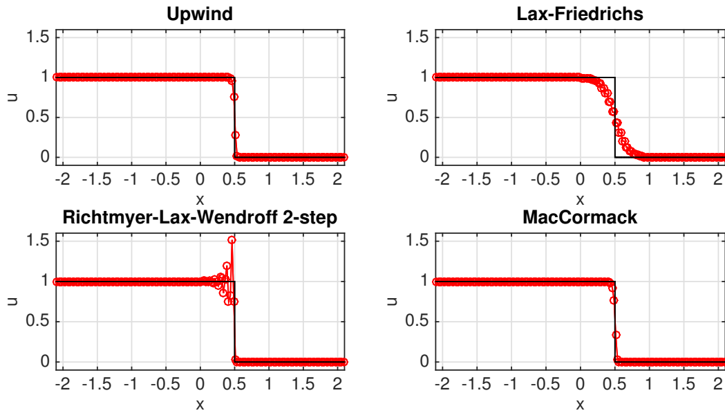
FIGURA 4.2. Ejemplo 4.2: solución numérica del problema de Riemann (4.10). La línea sólida es la solución exacta.
