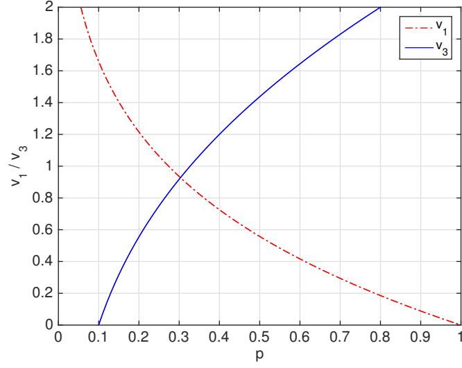
FIGURA 6.8. Ejemplo 6.12 (ecuaciones de Euler, problema de Sod): curvas v_1 y v_3 expresadas como función de p .
