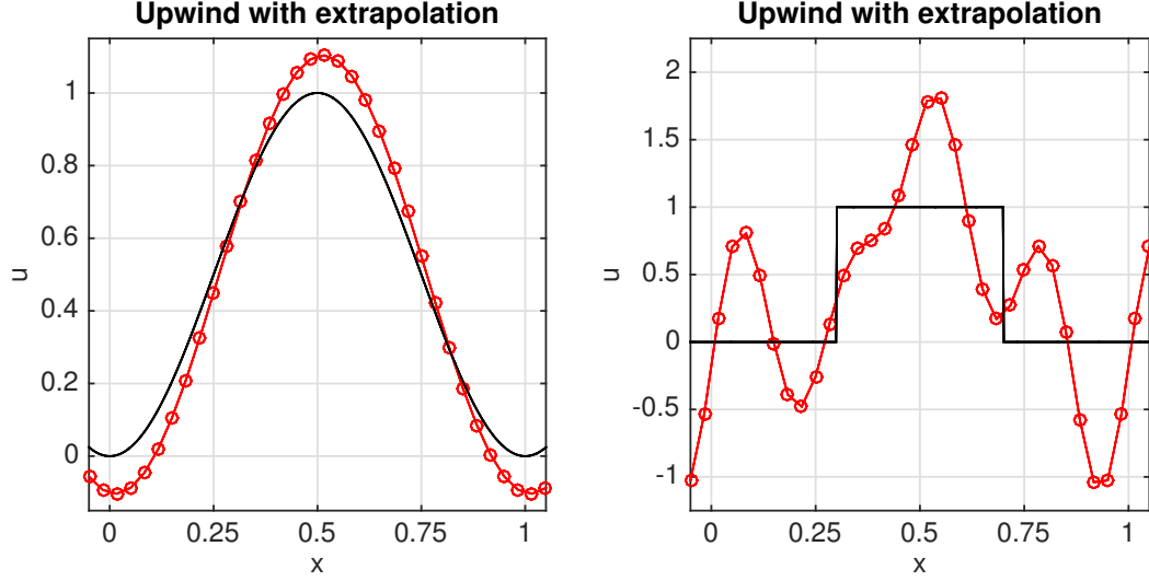
FIGURA 4.10. Ejemplo 4.8: solución de la ecuación de transporte u_t + u_x = 0 con el método upwind con extrapolación con dato inicial (izquierda) suave, (derecha) discontinuo constante a trozos.
