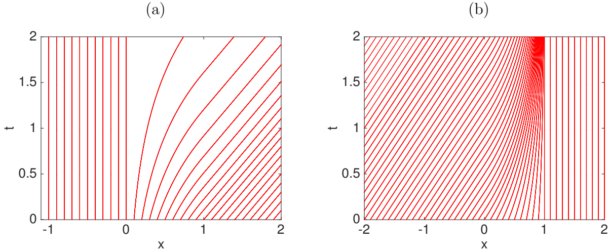
FIGURA 2.5. Ejemplos 2.10 y 2.11 (ecuación de transporte con coeficiente variable): características definidas (a) por (2.28) (Ejemplo 2.10), (b) por (2.29) (Ejemplo 2.11).
