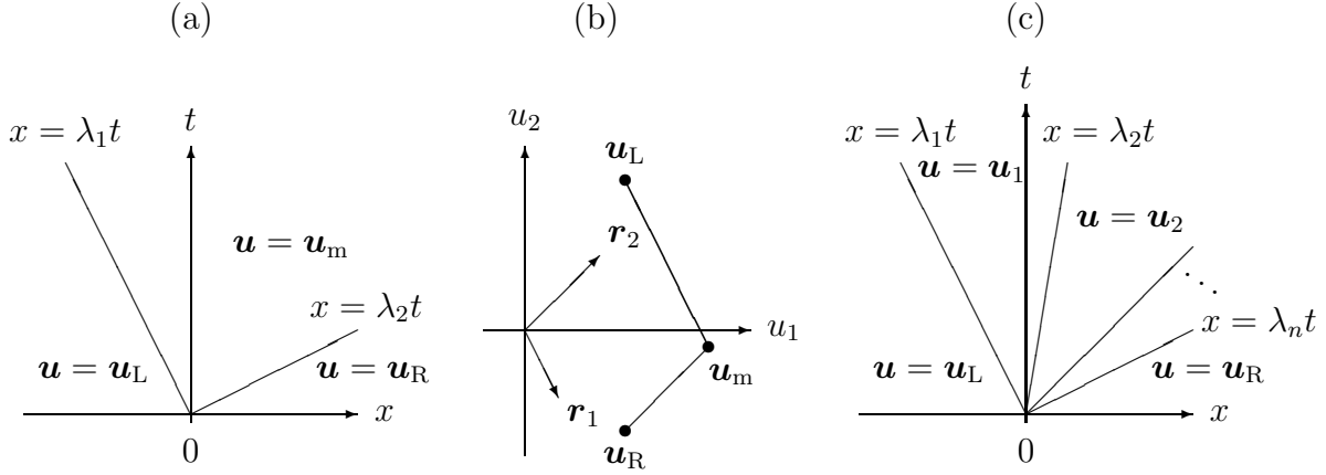
FIGURA 2.6. Solución del problema de Riemann para un sistema lineal: (a) solución (2.61) de un sistema de n = 2 ecuaciones, (b) construcción del estado intermedio \mathbf{u}_m en el espacio de fase, (c) solución (2.62) para n general.
