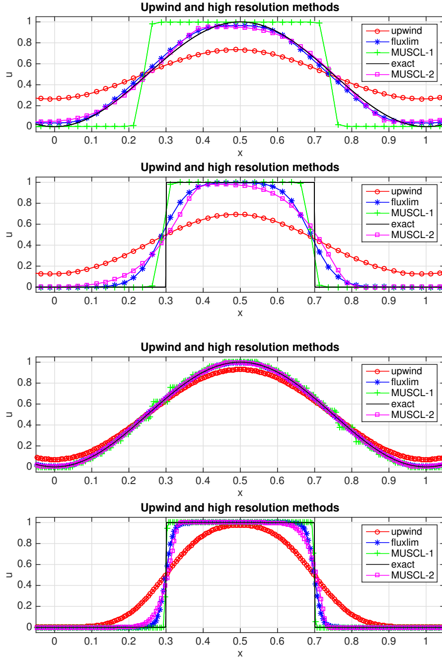
FIGURA 4.12. Ejemplo 4.9 (continuación): soluciones numéricas para \Delta x = 1/40 (arriba) y \Delta x = 1/200 (abajo).
