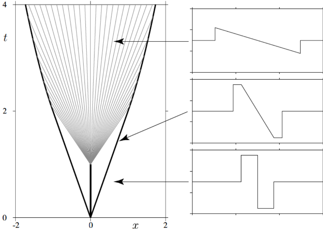
FIGURA 2.4. Ejemplo 2.8 (tráfico vehicular): solución del problema del semáforo en una carretera simple. Izquierda: solución en el plano (x, t) , derecha: solución u(x, t) en tres instantes t fijos.
